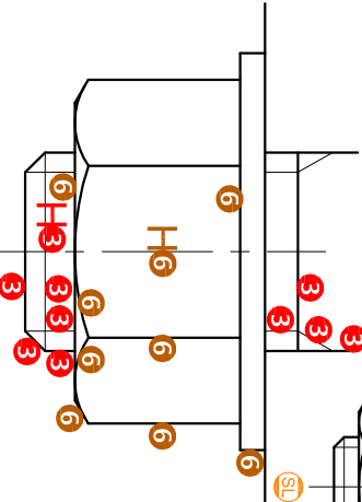
BESONDERHEDE VAN PUNTETOEKENNING VAN DIE WASTER, M12-MOER EN M12-BOUT
