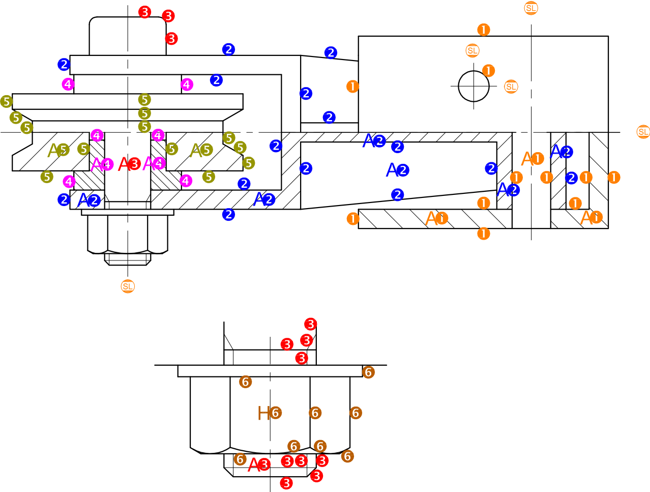
BESONDERHEDE VAN PUNTETOEKENNING VAN DIE WASTER, M12-MOER EN M12-BOUT
