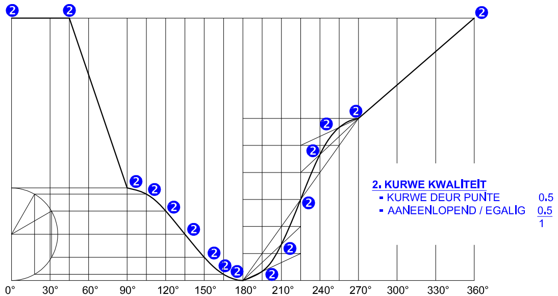
VERPLASINGSGRAFIK SKAAL 360° : 120 mm
