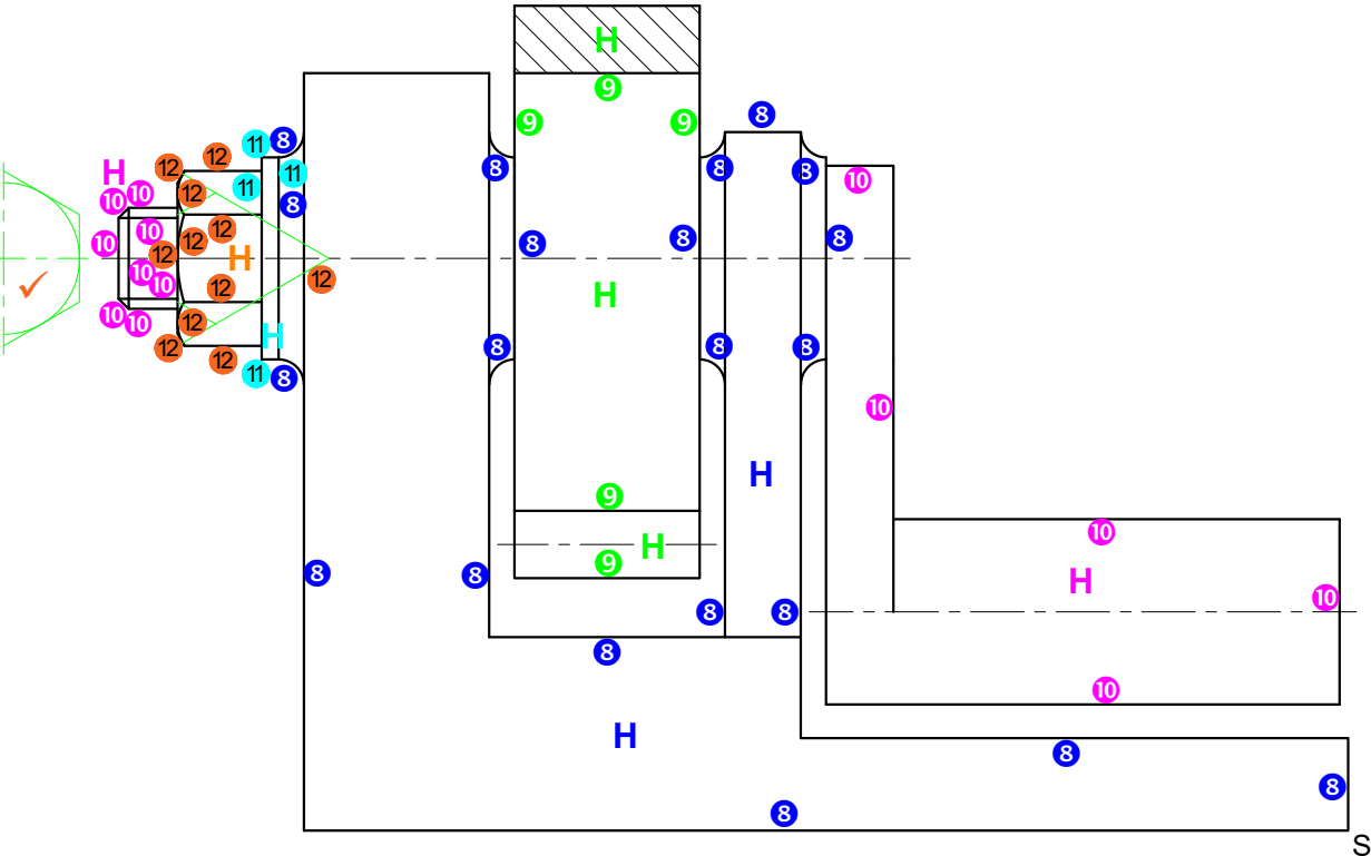
HALF SNIT VOORAANSIG 15 SKAAL 1 : 1 15
