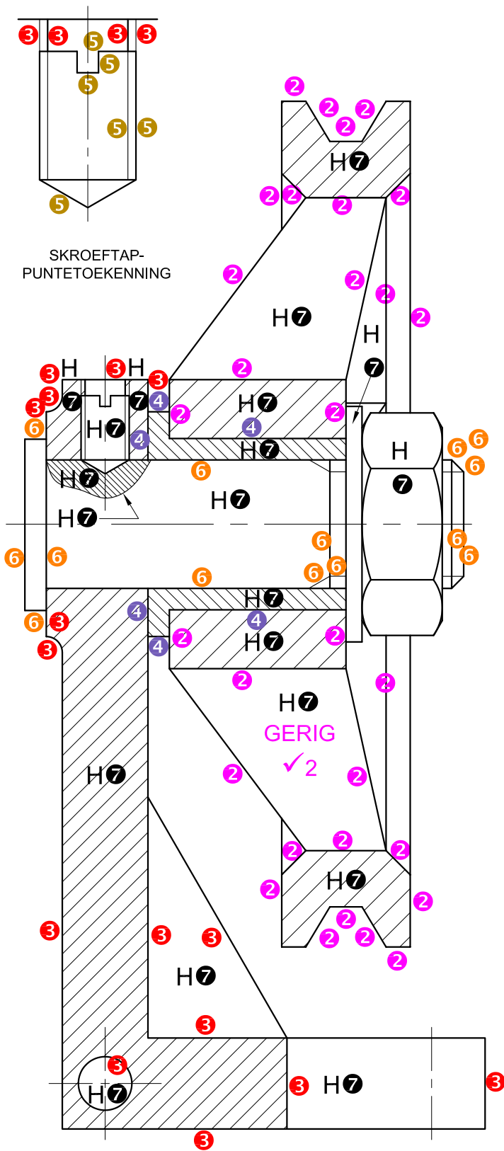
SNIT A-A 3
